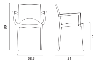
Dimensioni/Dimensions (cm.)
