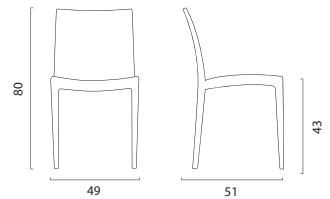
Dimensioni/Dimensions (cm.)
