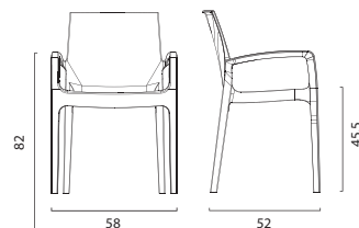
Dimensioni/Dimensions (cm.)
